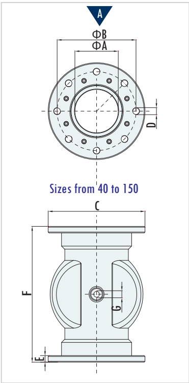
Pinch Valve 夹管阀
